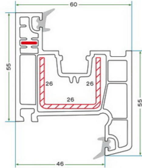
KYS 8003 KANAT PROFİLİ KYS 8003 SASH PROFILE
