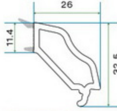
(KSR 009) 80'LIK ÜÇ CAM ÇİTASI (KSR 009) 80 TRIPLE WITH GRAY GASKET
