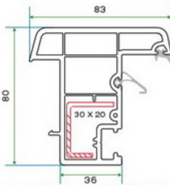
(KSR 007) 80'LİK HAREKETLİ ORTA KAYIT PROFİLİ (KSR 007) 80 MOVABLE MULLION PROFILE
