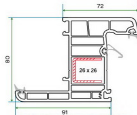
(KSR 004) 80'LİK PERVAZLI KASA PROFİLİ (KSR 004) FRAME PROFILE WITH BORDER
