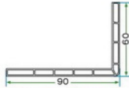
K 6024 60 x 90 PERVAZLI PROFİLİ K 6024 60 x 90 BORDER PROFILE
