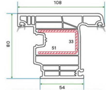
(KSR 006) 80'LİK DIŞA AÇILIR KAPI PROFİLİ (KSR 006) 80 OUTWARD OPENING DOOR SASH PROFILE
