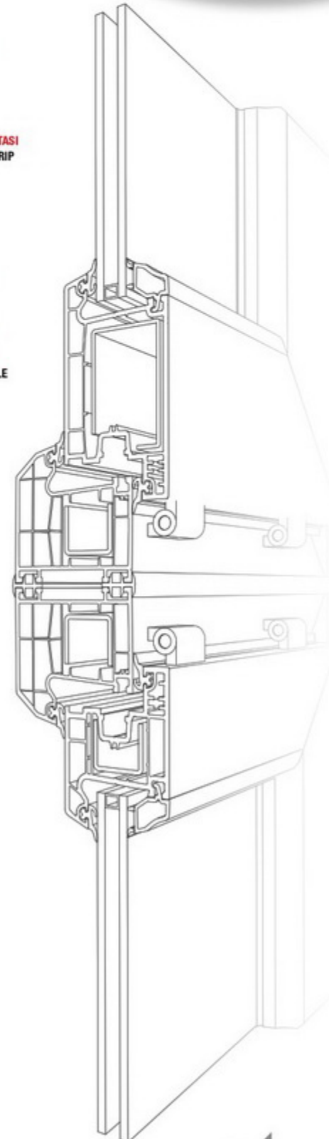
K 6013 BAĞ PROFİLİ K 6013 COUPLING PROFILE
