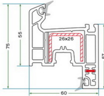
K 6004 KANAT PROFİLİ K 6004 SASH PROFILE
