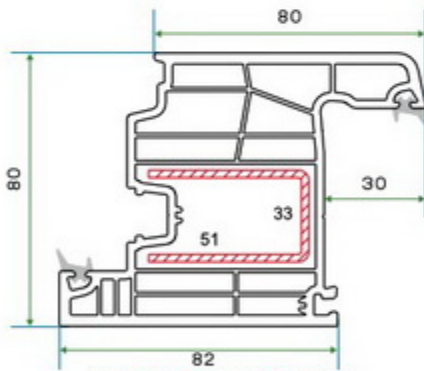
(KSR 005) 80'LİK KAPI PROFİLİ (KSR 005) 80 DOOR PROFILE
