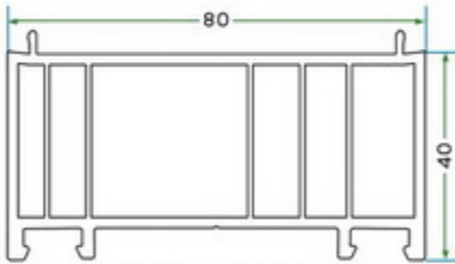
KSR 010 80'LIK KASA YÜKSELTME APARATI K 6025 DRAIN CLOSING STRIP
