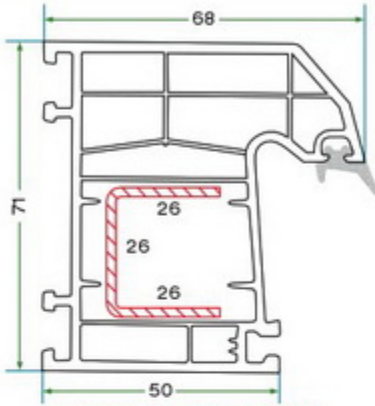
KKS 005 SÜPER KASA PROFİLİ KKS 005 SUPER FRAME PROFILE
