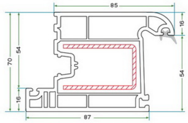
KRS 004 70'LİK KAPI PROFİLİ KRS 004 70 DOOR SASH PROFILE
