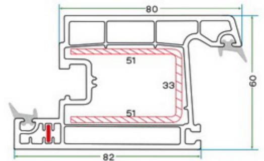
K 6022 BALKON KAPI KANAT PROFİLİ K 6022 BALCONY DOOR SASH PROFILE
