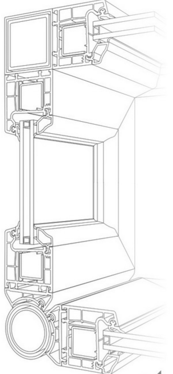
K 6025 KANAL KAPATMA ÇİTASI K 6025 DRAIN CLOSING STRIP
