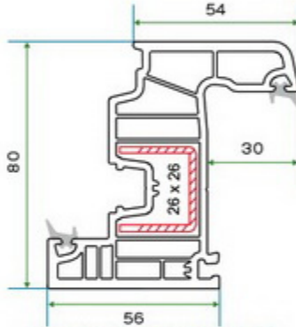
(KSR 003) 80'LİK KANAT PROFİLİ (KSR 003) 80 SASH PROFILE
