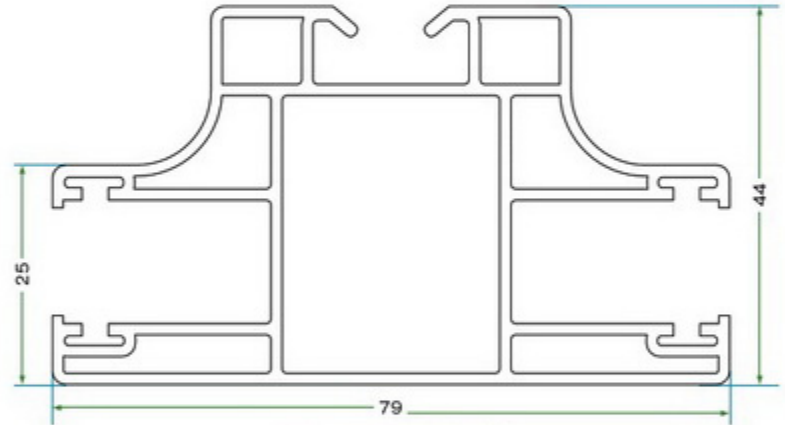
KMS 007 ORTA KAYIT PROFİLİ KMS 007 ORTA KAYIT PROFİLİ
