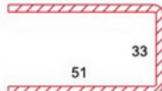
DIŞA AÇILIR KAPI PROFİLİ DESTEK SAÇI OUTWARD DOOR STEEL REINFORCEMENT
