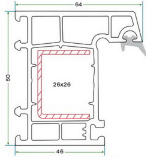
KYS 8004 46'LİK KASA PROFİLİ KYS 8004 46 FRAME PROFILE
