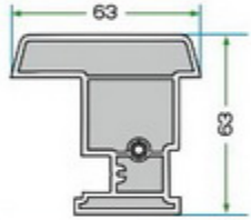
K 6023 HAR. ORTA KAYIT KAPAĞI K 6023 MOVABLE MULLION LID
