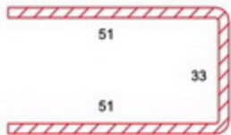
DIŞA AÇILIR KAPI DESTEK SAÇI OUTWARD OPENING DOOR STEEL REINFORCEMENT
