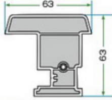
K 6023 HAREKETLİ ORTA KAYIT KAPAĞI K 6023 MOVABLE MULLION LID
