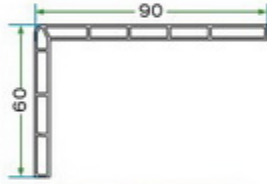
K 6024 60 x 90 PERVAZ PROFİLİ K 6024 60 x 90 BORDER PROFILE
