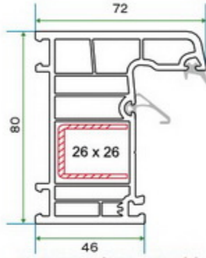
(KSR 001) 80'LİK KASA PROFİLİ (KSR 001) 80 FRAME PROFILE
