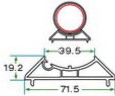
KKS 006 70 mm KÖŞE DÖNÜŞ ADAPTÖRÜ KKS 006 70 mm CORNER ADAPTER
