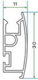
KMS 006 PANJUR ÇİTASI KMS 006 PANJUR ÇİTASI
