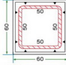
6 6009 60 x 60 KUTU PROFİLİ K 6009 60 x 60 BOX PROFILE
