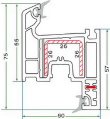
K 6004 KANAT PROFİLİ K 6004 SASH PROFILE
