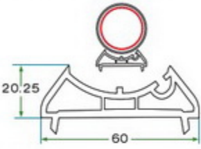
K 6011 60 mm KÖŞE DÖNÜŞ ADAPTÖRÜ K 6011 60 mm CORNER ADAPTER
