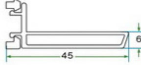
K 6015 ÇAKMA PERVAZ PROFİLİ K 6015 NAILING BORDER PROFILE
