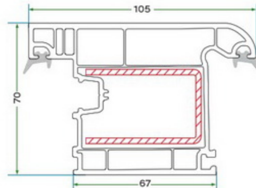
KRS 010 70'LİK DIŞA AÇILIR KAPI PROFİLİ KRS 010 OUTWARD OPENING DOOR SASH PROFILE
