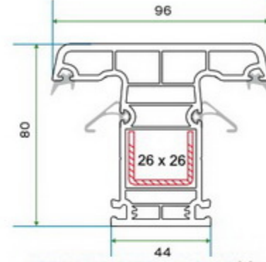
(KSR 002) 80'LİK ORTA KAYIT PROFİLİ (KSR 002) 80 MULLION PROFILE
