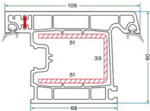
K 6016 DIŞA AÇILIR KAPI KANAT PROFİLİ K 6016 OUTWARD OPENING DOOR SASH PROFILE
