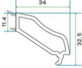
(KSR 008) 80'LIK ÇİFT CAM ÇİTASI (KSR 008) 80 DOUBLE WITH GRAY GASKET
