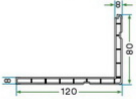
K 6010 80 x 120 PERVAZ PROFİLİ K 6010 80 x 120 BORDER PROFILE
